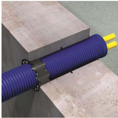
Figure 1 - Tubes préisolés Microflex
