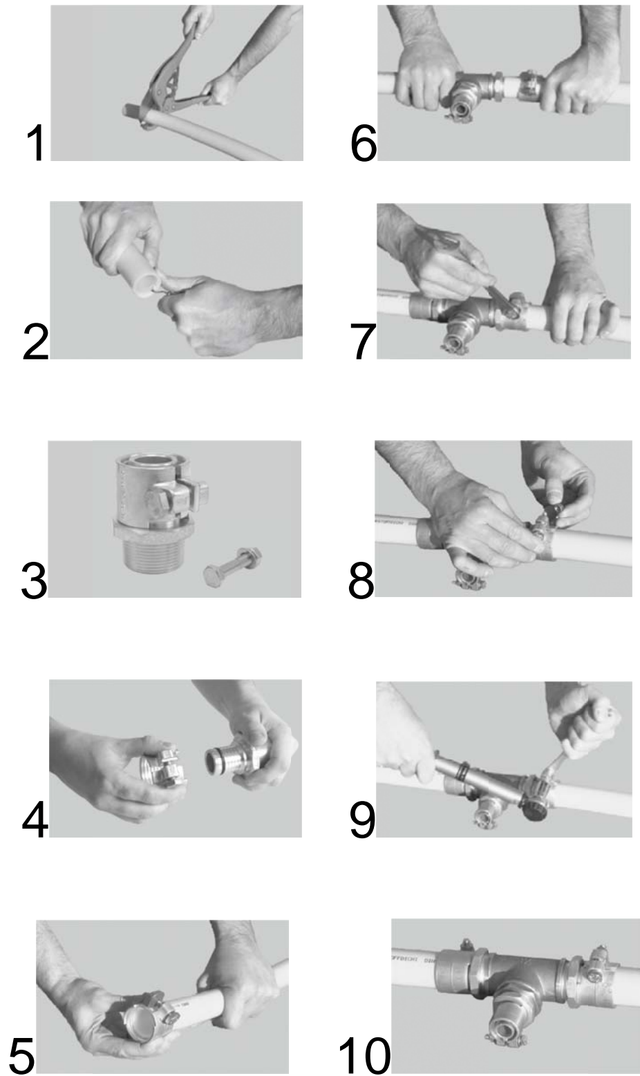
Figure 1 - Réalisation des assemblages
